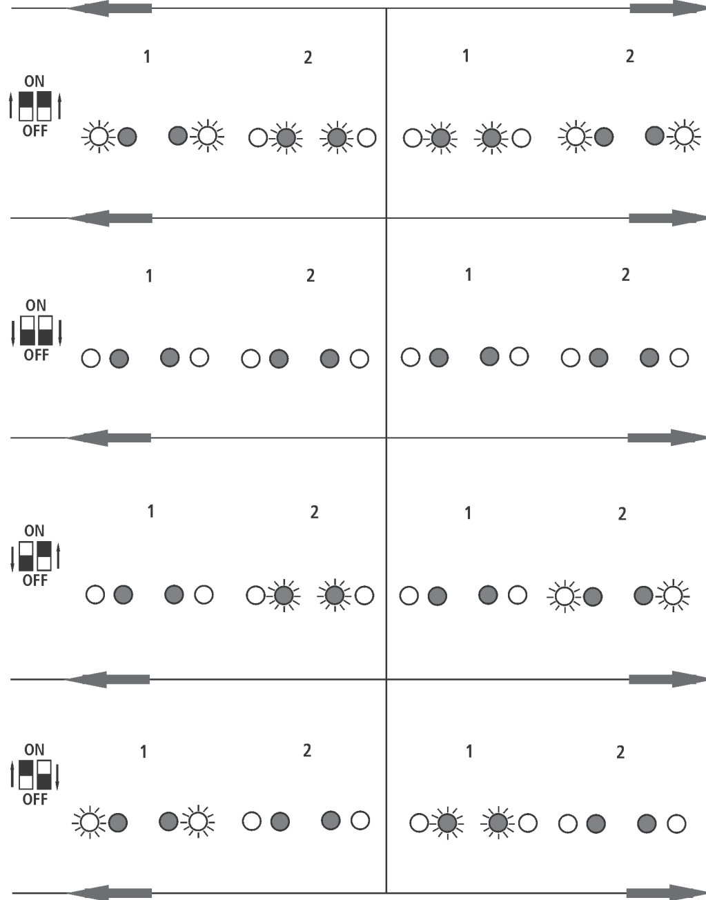
Fig. 5 Fahrtrichtung Direction
